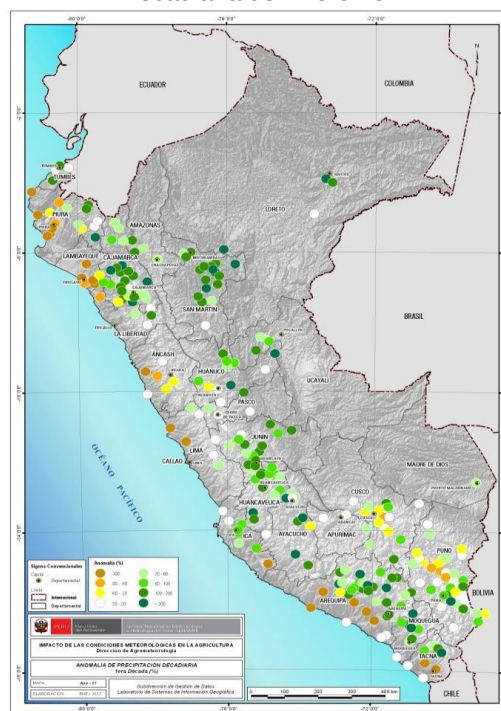
Figura 2: Anomalías de precipitación (%) 1° Decadiaria de Enero 2017
