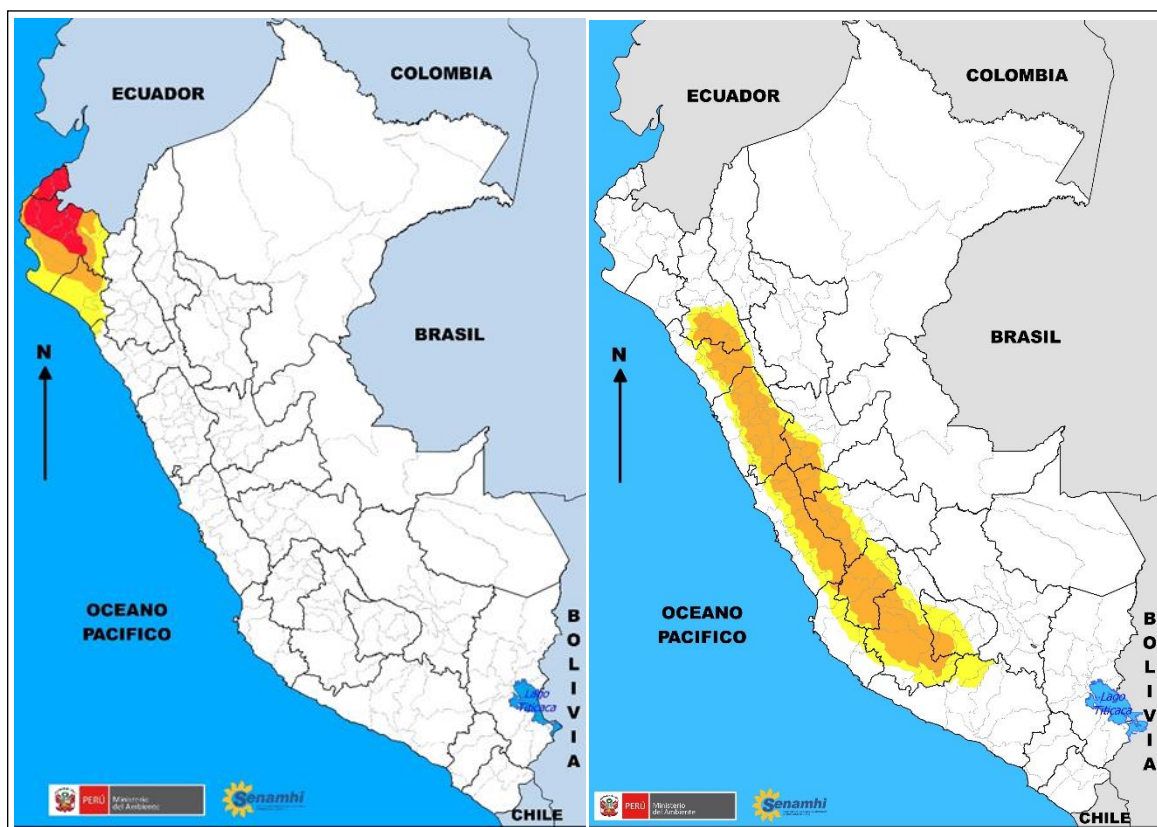
Figura 4: Pronóstico de lluvias para el periodo del 30 de enero al 06 de Febrero 2017.
