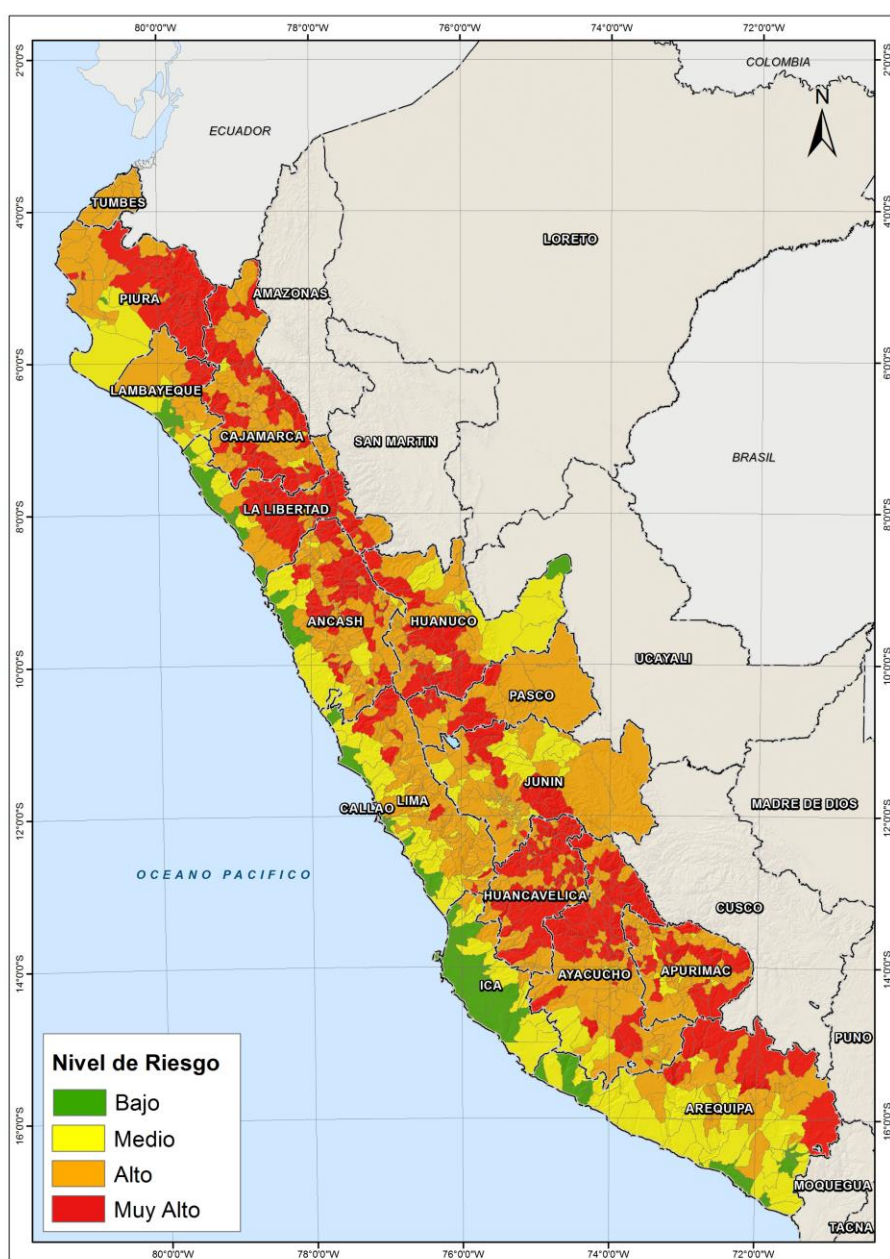
Figura N° 5: Escenario de riesgo por movimientos en masa ante el pronóstico de precipitación para el periodo del 02 al 04 de Febrero de 2017
