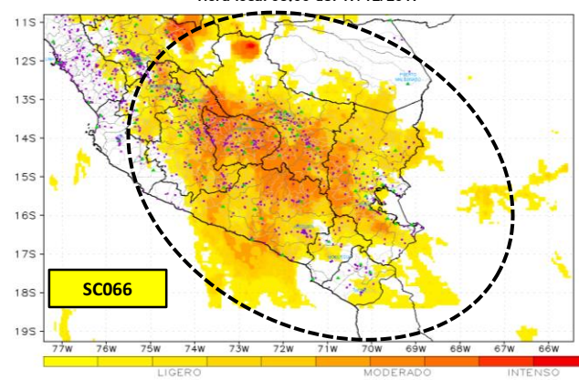
PRONÓSTICO DE AREA DE MAL TIEMPO Hora local 08:00 del 17/12/2017
