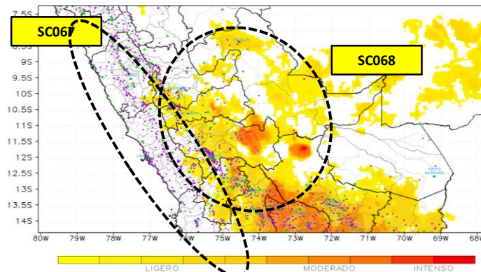
PRONÓSTICO DE AREA DE MAL TIEMPO Hora local 08:00 del 17/12/2017
