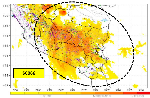
PRONÓSTICO DE AREA DE MAL TIEMPO Hora local 06:00 del 17/12/2017
