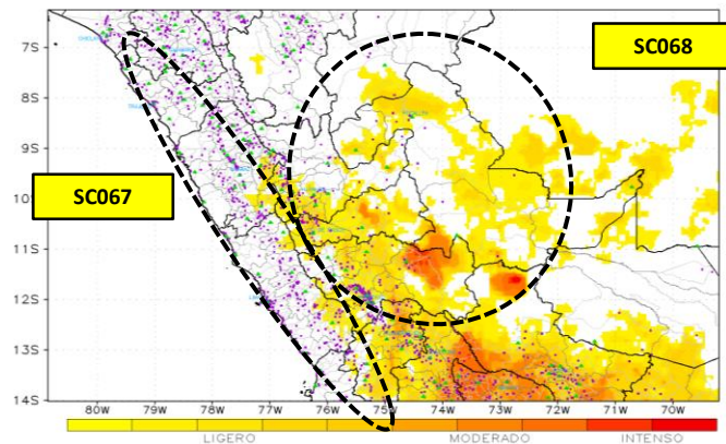
PRONÓSTICO DE AREA DE MAL TIEMPO Hora local 06:00 del 17/12/2017
