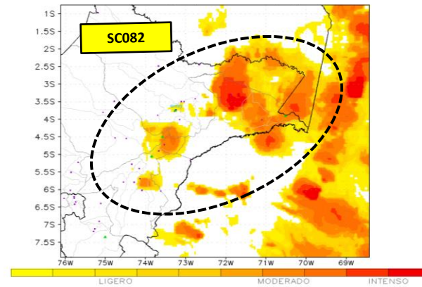
PRONÓSTICO DE AREA DE MAL TIEMPO Hora local 22:00 del 18/12/2017
