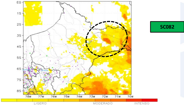
PRONÓSTICO DE AREA DE MAL TIEMPO Hora local 08:00 del 19/12/2017
