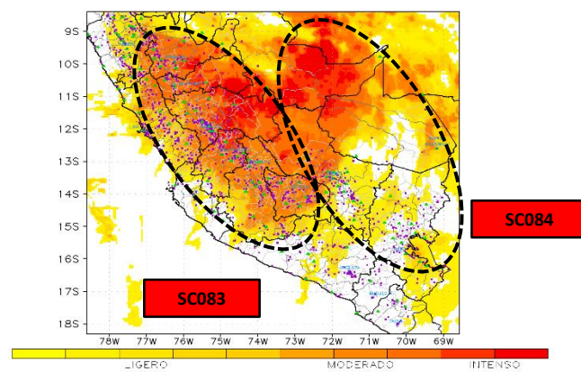
PRONÓSTICO DE AREA DE MAL TIEMPO Hora local 08:00 del 19/12/2017
