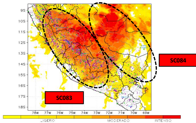
PRONÓSTICO DE AREA DE MAL TIEMPO Hora local 06:00 del 19/12/2017
