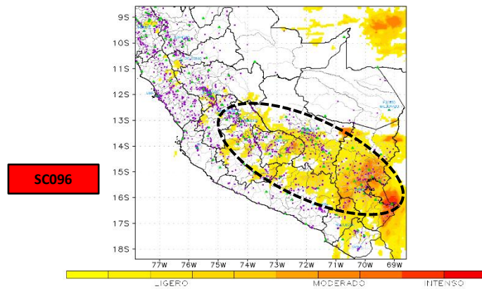
PRONÓSTICO DE AREA DE MAL TIEMPO Hora local 22:15 del 22/12/2017
