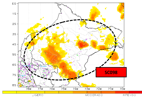
PRONÓSTICO DE AREA DE MAL TIEMPO Hora local 22:15 del 22/12/2017
