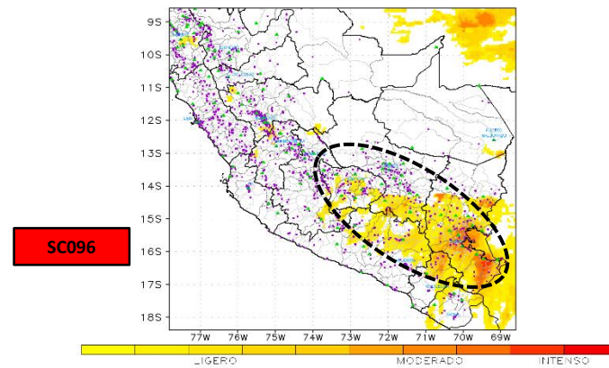
PRONÓSTICO DE AREA DE MAL TIEMPO Hora local 00:15 del 23/12/2017
