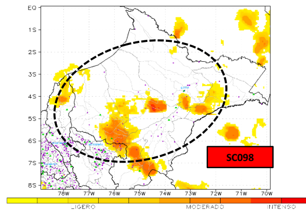
PRONÓSTICO DE AREA DE MAL TIEMPO Hora local 00:15 del 23/12/2017
